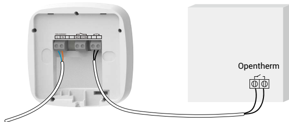
Schéma de câblage de la chaudière Opentherm
