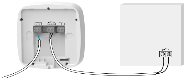
Schéma de câblage marche/arrêt de la chaudière
